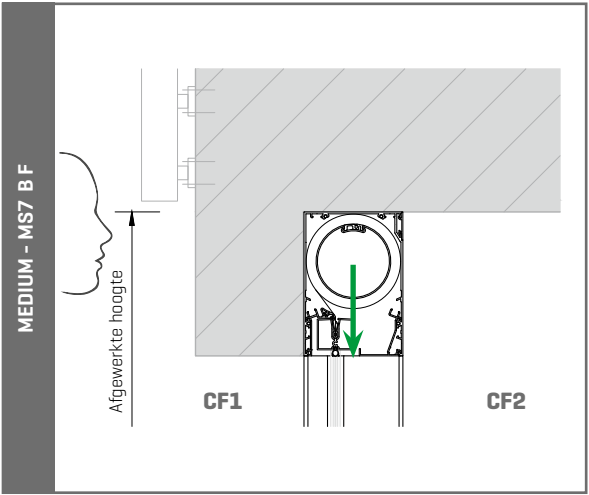
Richting uitneembaarheid doekset
