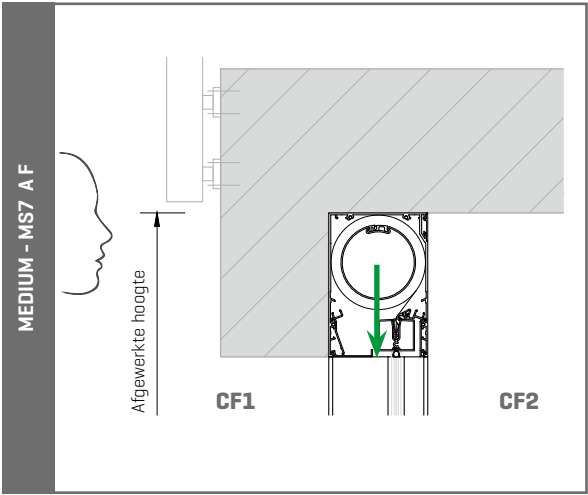
Kijkrichting bepaalt keuzeoptie kabeldoorvoer links of rechts
