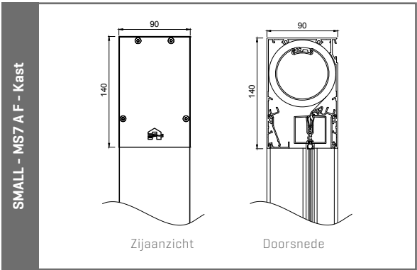
Kijkrichting bepaalt keuzeoptie kabeldoorvoer links of rechts
